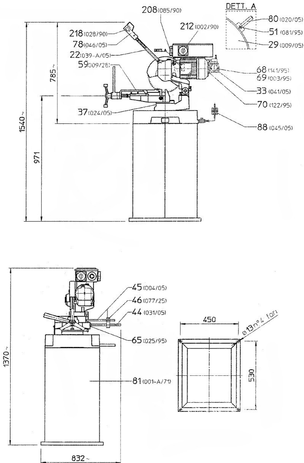
Abb./ Fig. 1: Ersatzteilzeichnung 1 - MKS 250 N/MKS 255 N / Spare parts drawing 1 - MKS 250 N/MKS 255 N
