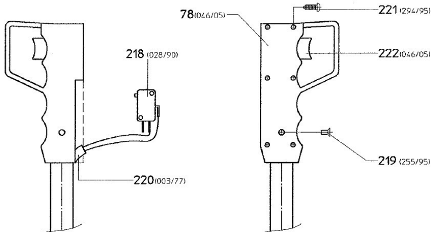
Abb. / Fig. 3: Ersatzteilzeichnung 3 - MKS 250 N/MKS 255 N / Spare parts drawing 3 - MKS 250 N/MKS 255 N
