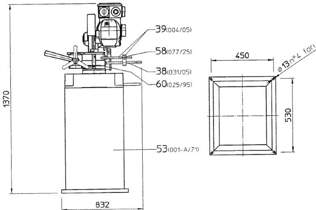
Abb. / Fig. 5: Ersatzteilzeichnung 1 - MKS 275 N / Spare parts drawing 1 - MKS 275 N
