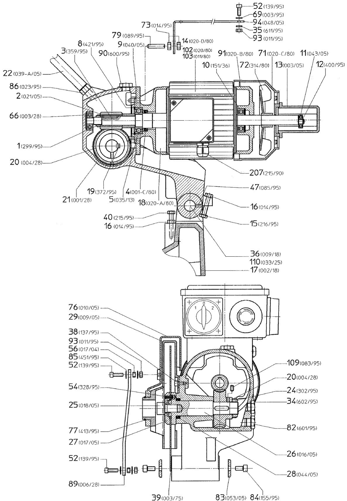
Abb. / Fig 2: Ersatzteilzeichnung 2 - MKS 250 N/MKS 255 N / Spare parts drawing 2 - MKS 250 N/MKS 255 N
