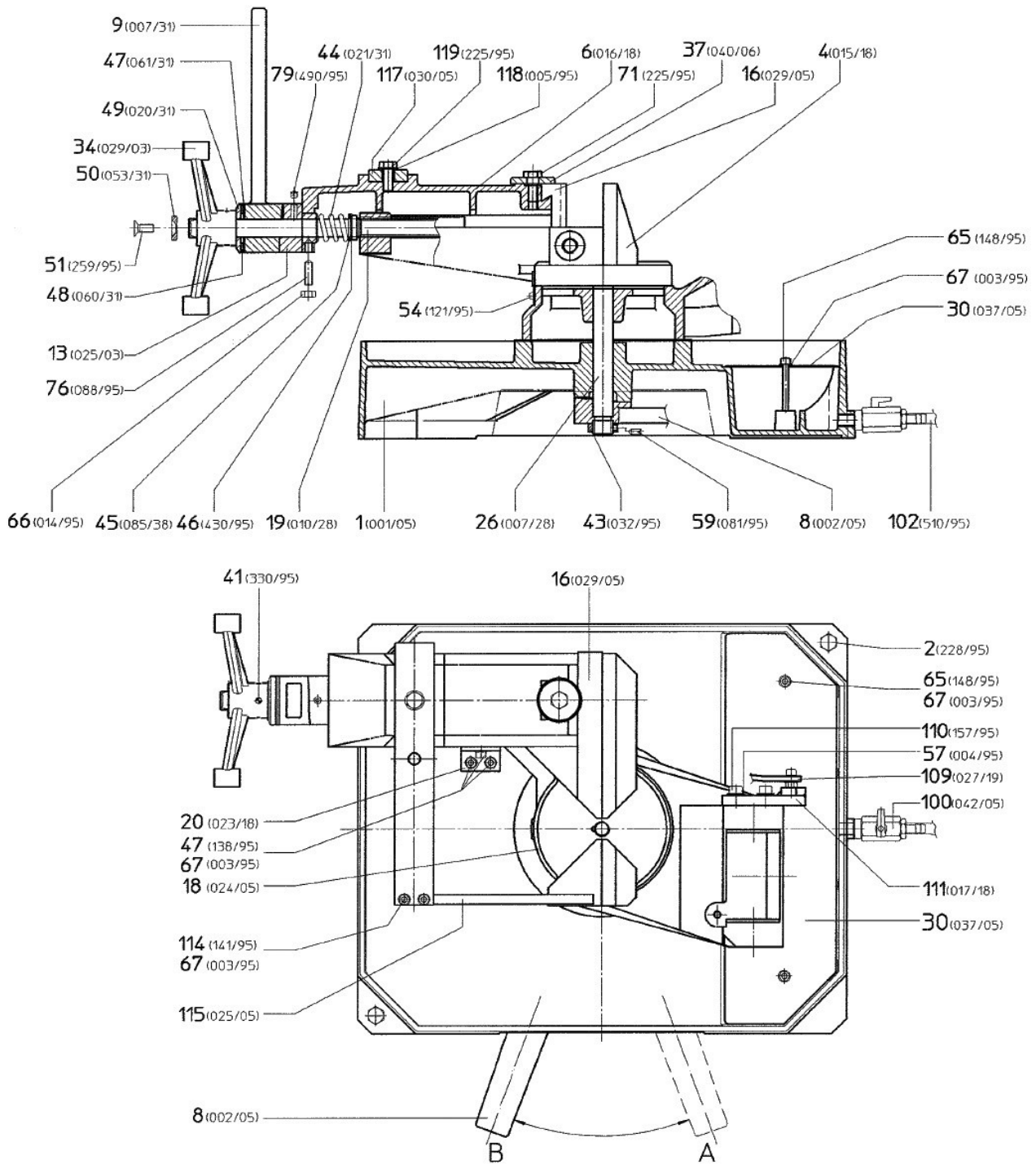
Abb. / Fig. 7: Ersatzteilzeichnung 3 - MKS 275 N / Spare parts drawing 3 - MKS 275 N
