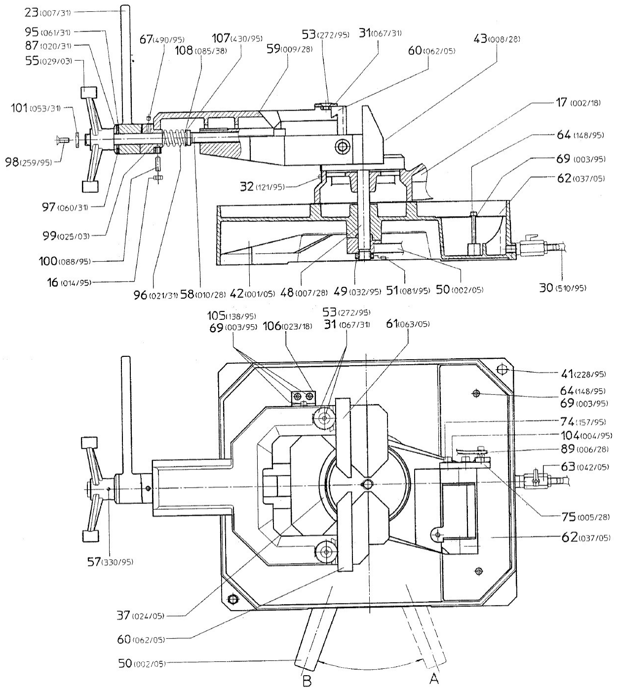
Abb. / Fig. 4: Ersatzteilzeichnung 4 - MKS 250 N/MKS 255 N / Spare parts drawing 4 - MKS 250 N/MKS 255 N
