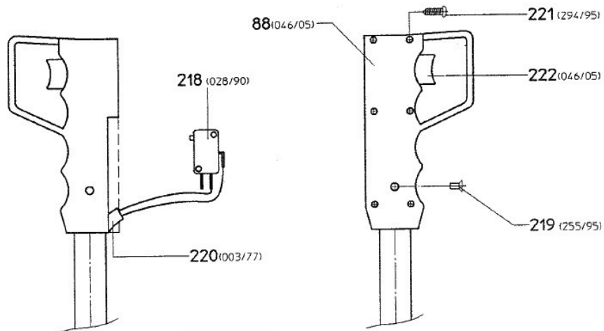
Abb. / Fig. 8: Ersatzteilzeichnung 4 - MKS 275 N / Spare parts drawing 4 - MKS 275 N
