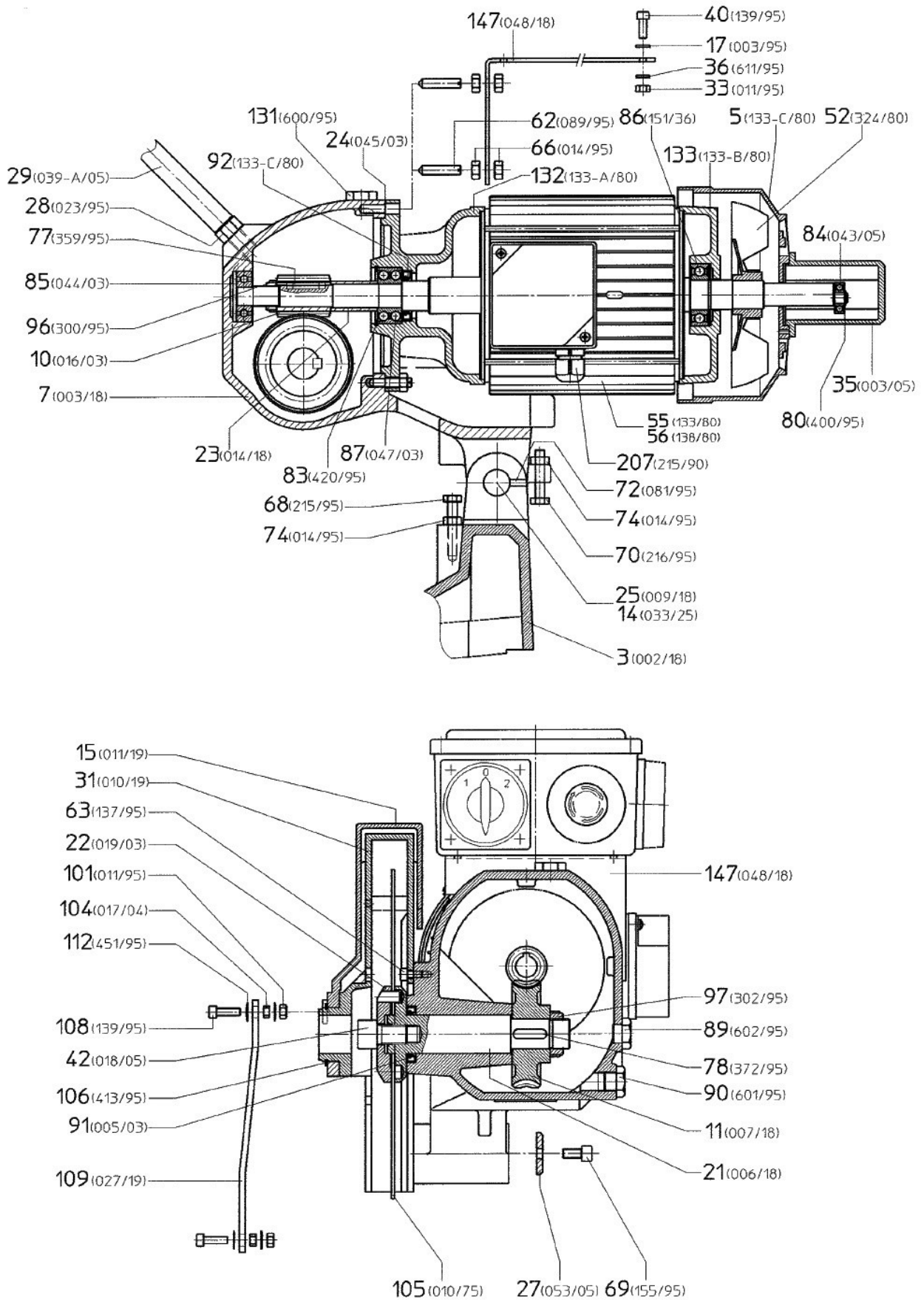
Abb. / Fig. 6: Ersatzteilzeichnung 2 - MKS 275 N / Spare parts drawing 2 - MKS 275 N
