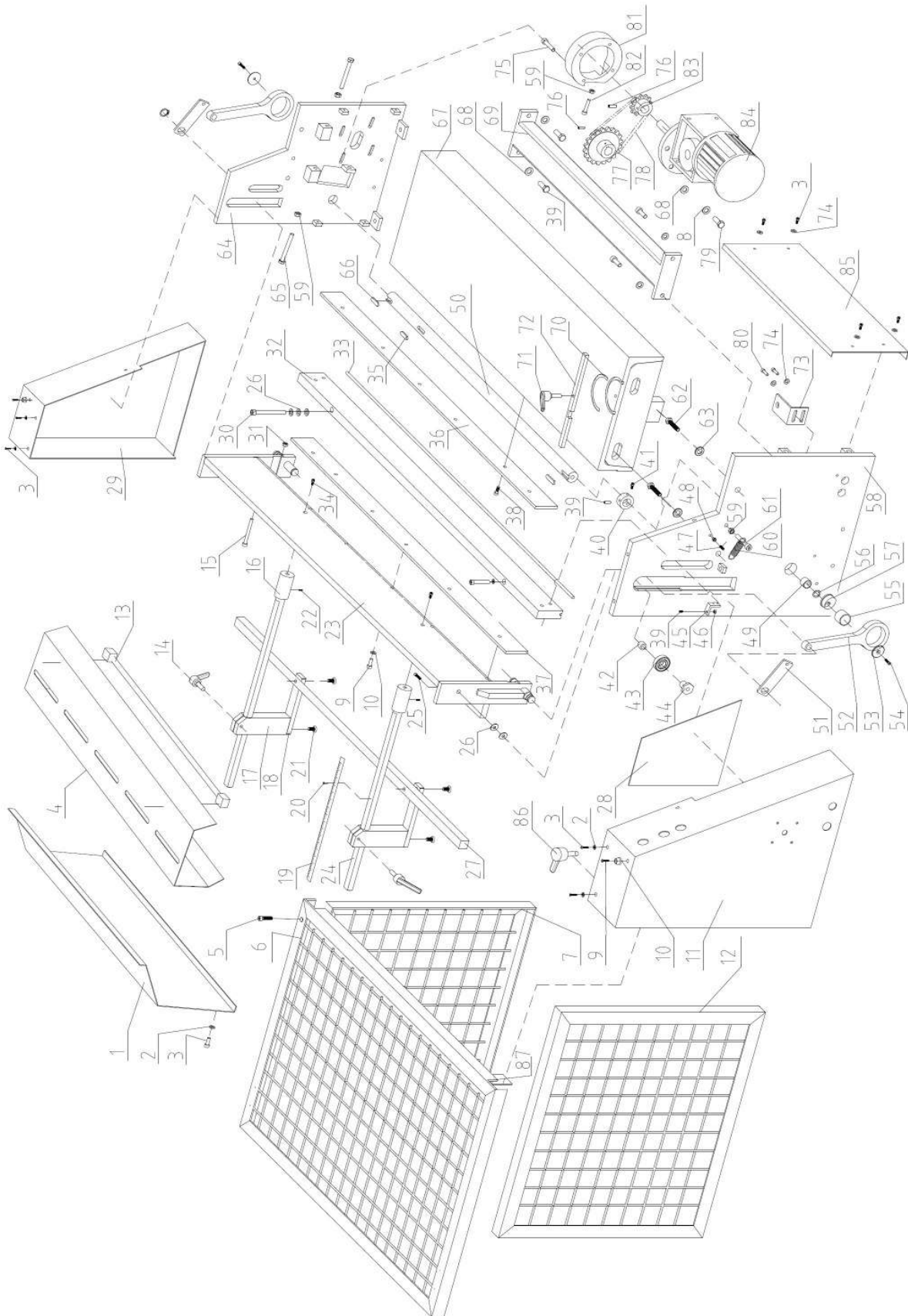
Abb. / Fig. 1: Ersatzteilzeichnung / Spare parts drawing
