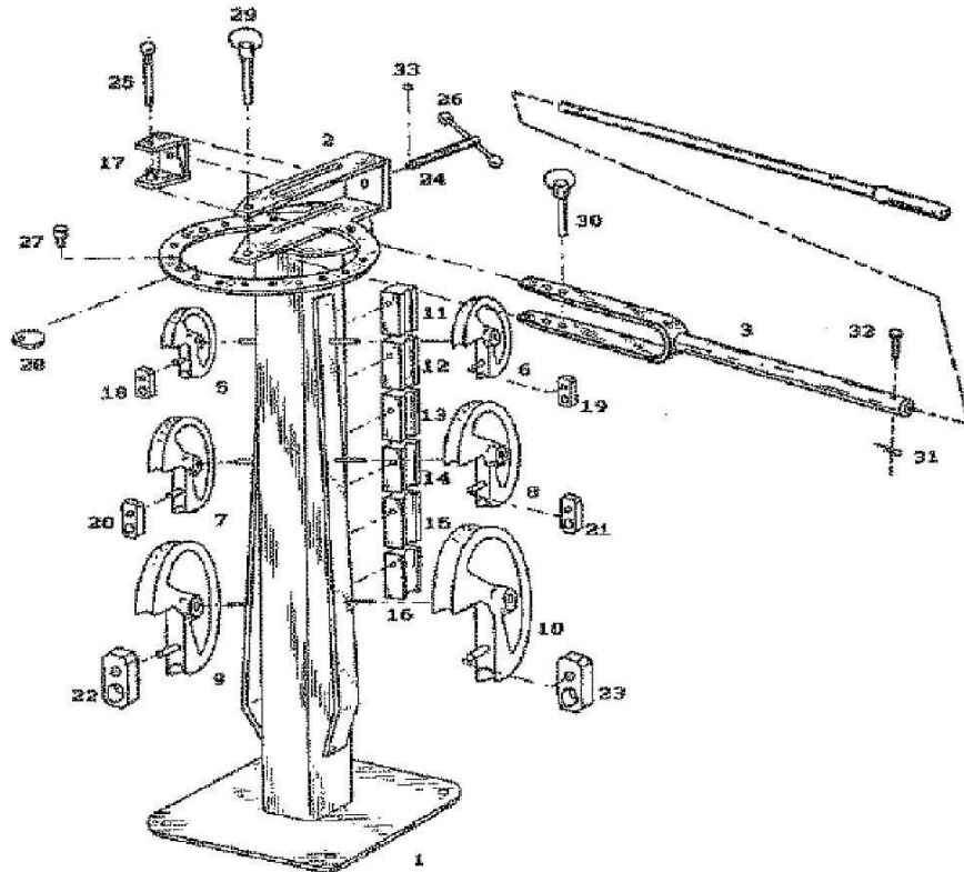
Abb. / Fig. 1: Ersatzteilzeichnung 1 / Spare parts drawing 1 (RB 30)
